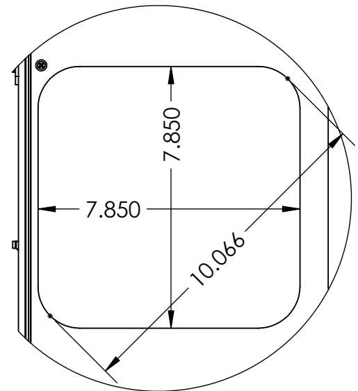
Cutout Dimensions
