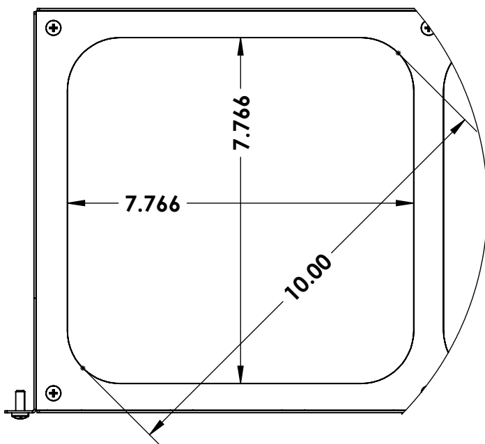
Cutout Dimensions
